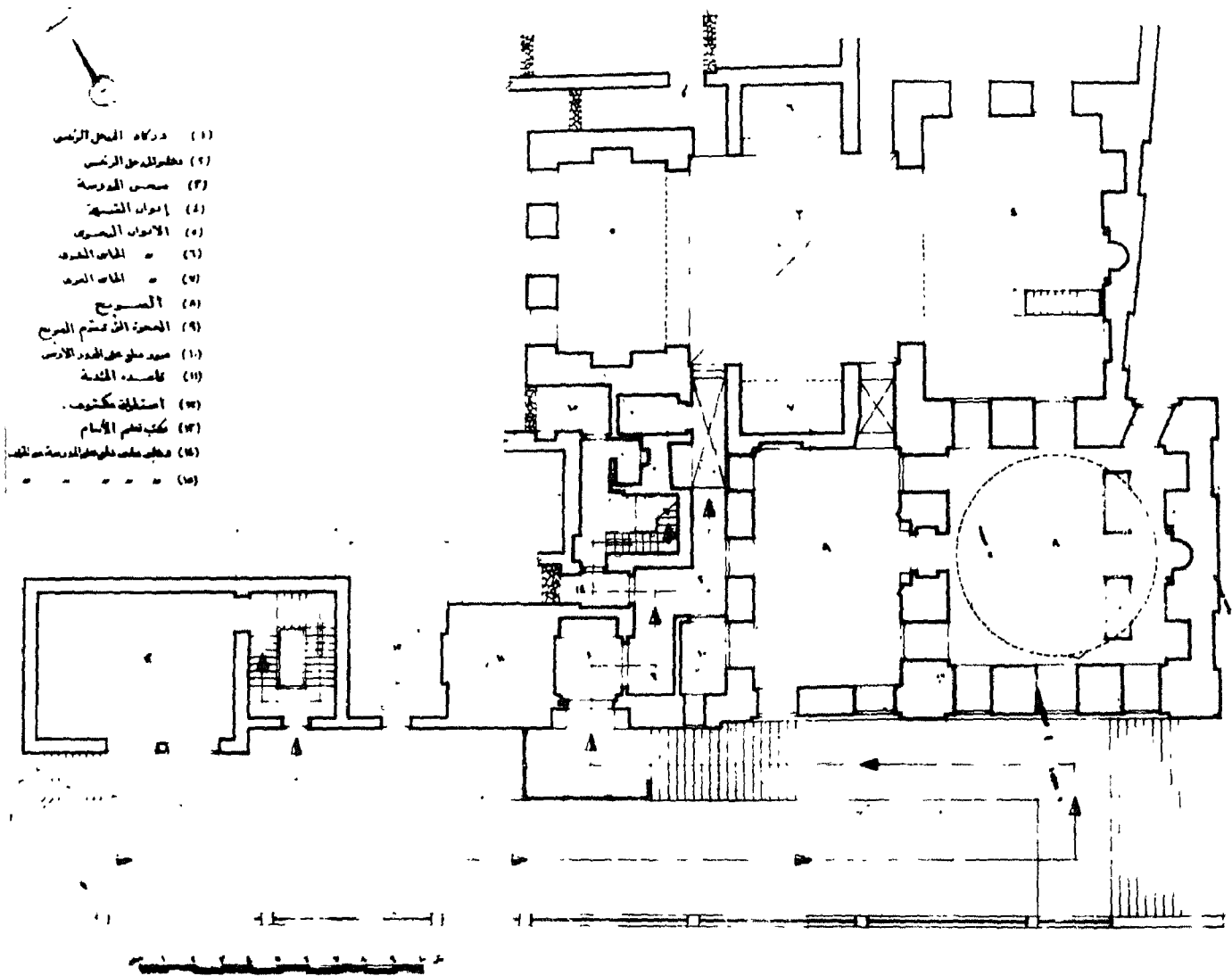
شكل (١٦) يبين مسقط أفقى لمدرسة قناني باي الرماح بميدان القلعة (صلاح الدين حالياً)
